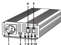
Панель переменного тока
