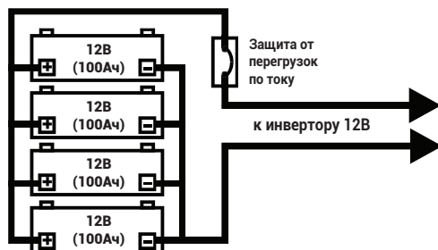
Блок аккумуляторов на 12 В (общая емкость = 400 Ач)
