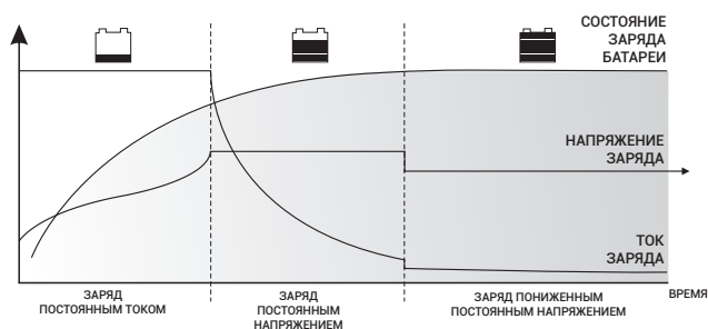
График этапов заряда аккумулятора
